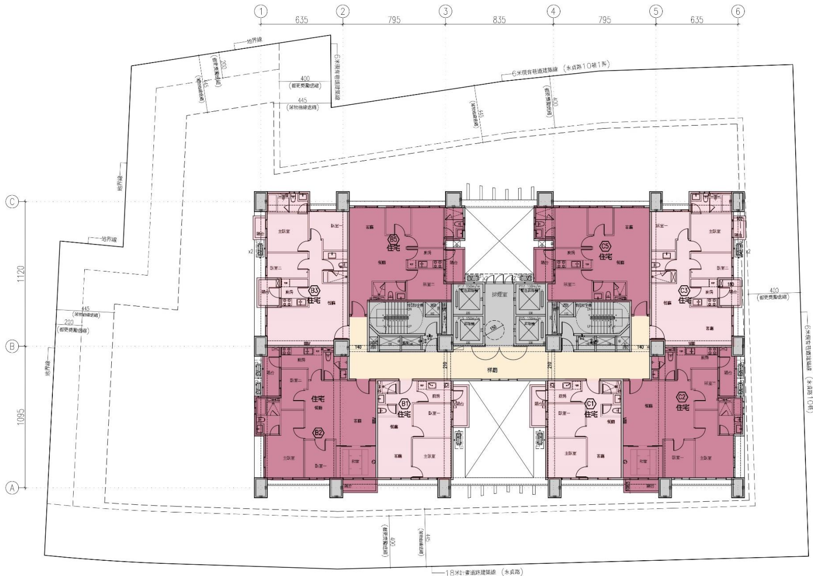
四至二十二層平面圖 S:1/200
