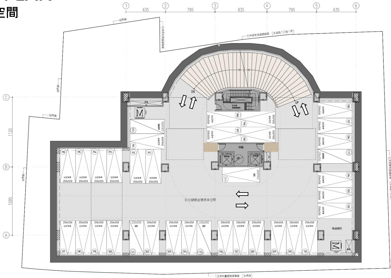
地下三層平面圖 S:1/200
