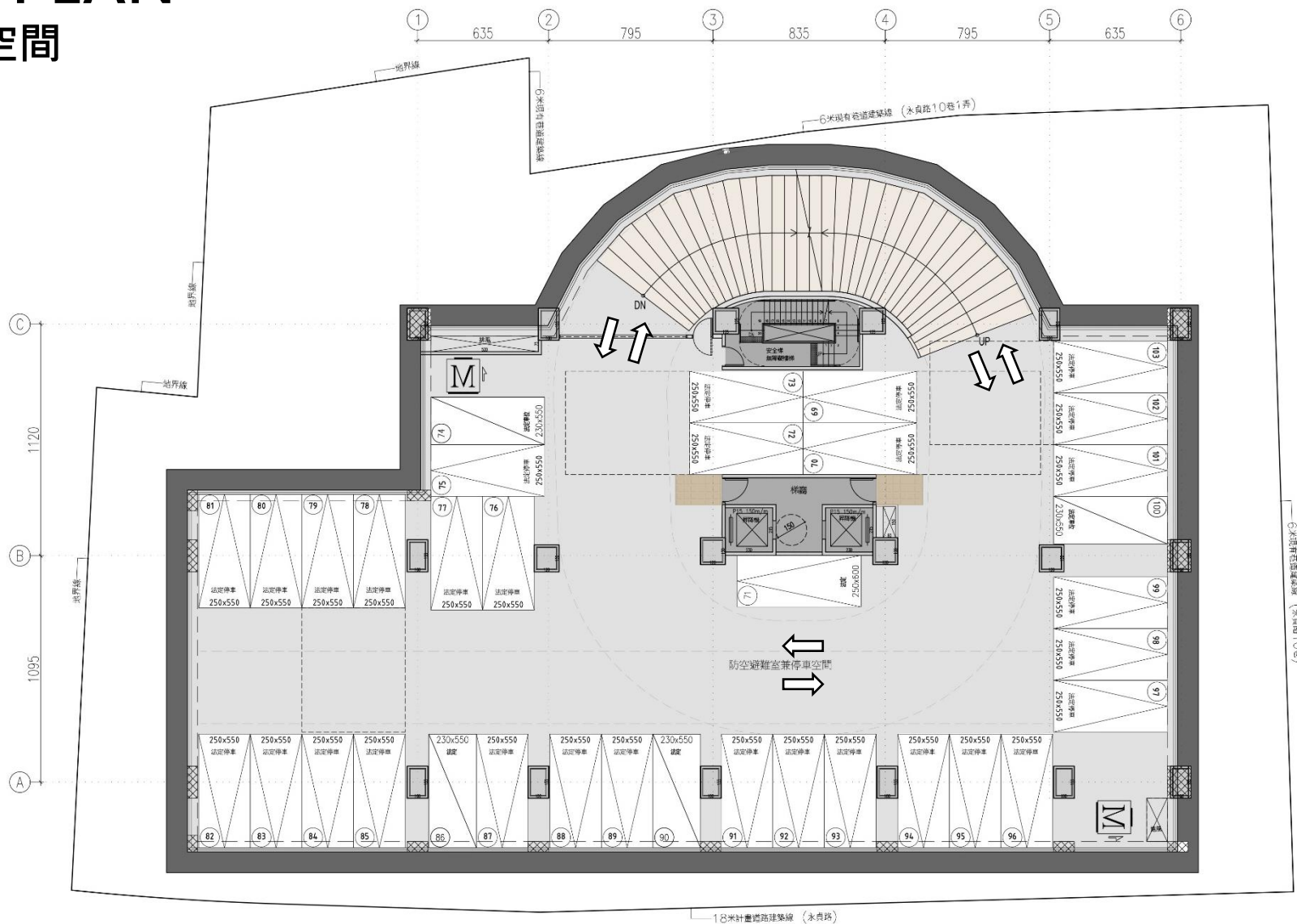
地下四層平面圖 S:1/200
