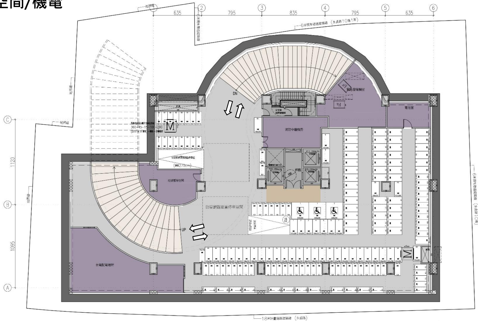
地下一層平面圖 S:1/200
