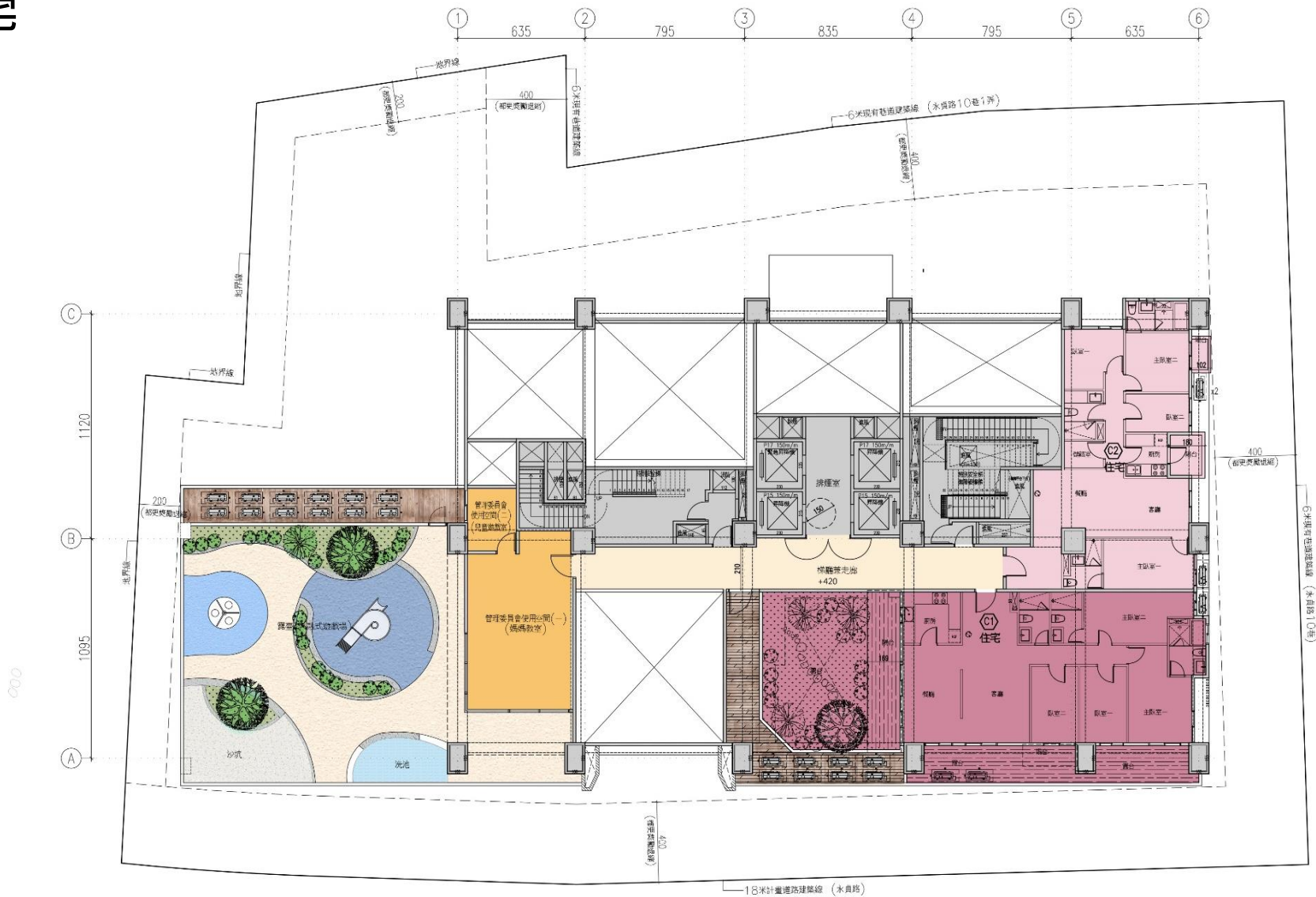
二層平面圖 S:1/200
