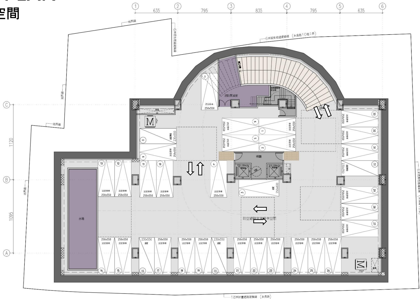
地下六層平面圖 S:1/200
