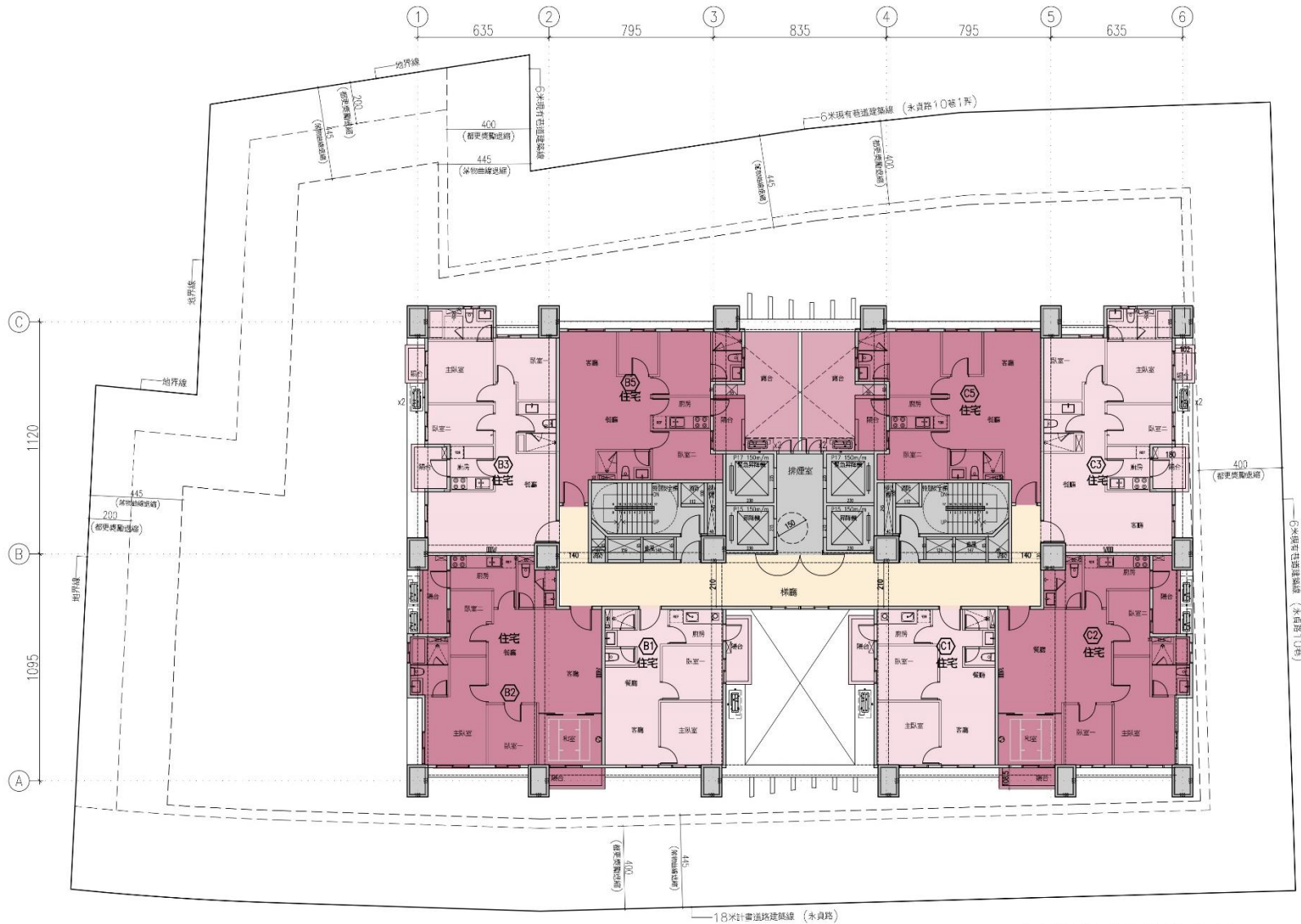
三層平面圖 S:1/200
